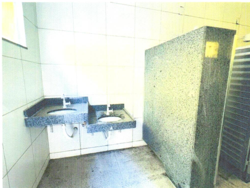
FOTO 44 – INSTALAÇÃO DE LAVATÓRIO COM BANCADA EM GRANITO CINZA ANDORINHA COM DUAS CUBAS DE EMBUTIR DE LOUÇA, SIFÃO CROMADO, VÁLVULA CROMADA E TORNEIRA CROMADA.
