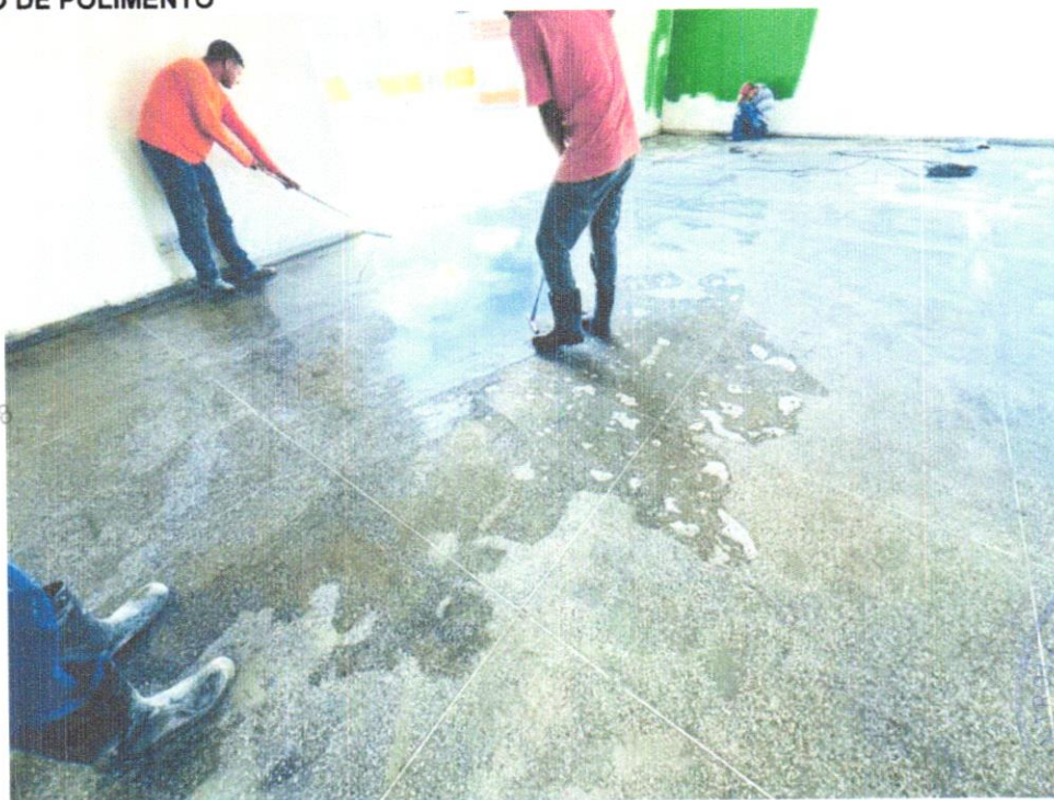
FOTO 28 – APLICAÇÃO DE PISO ALTA RESISTÊNCIA, COR CINZA, APLICADO COM JUNTAS E COM APLICAÇÃO DE POLIMENTO
